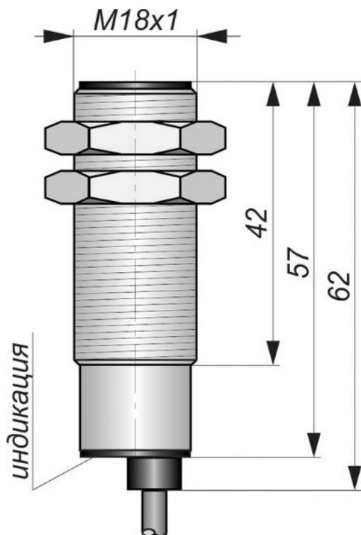
Габаритный чертеж
