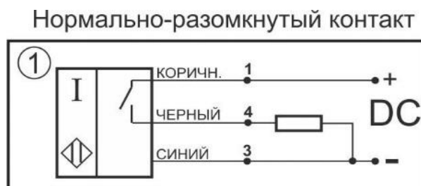
Схема соединения
