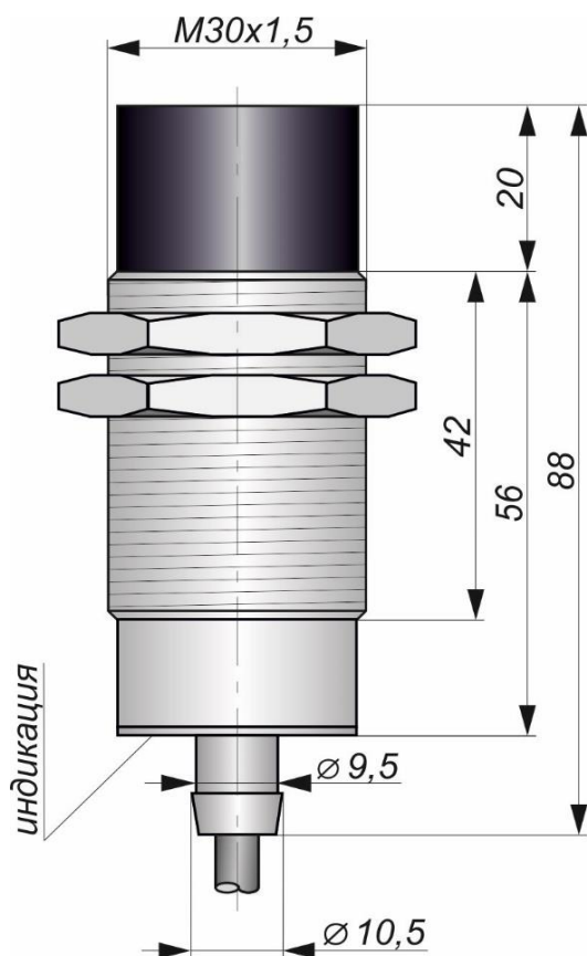
Габаритный чертеж
