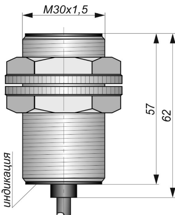
Габаритный чертеж
