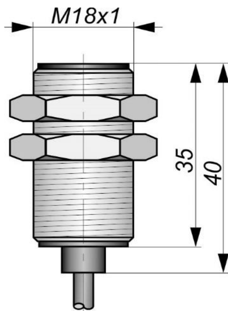
Габаритный чертеж
