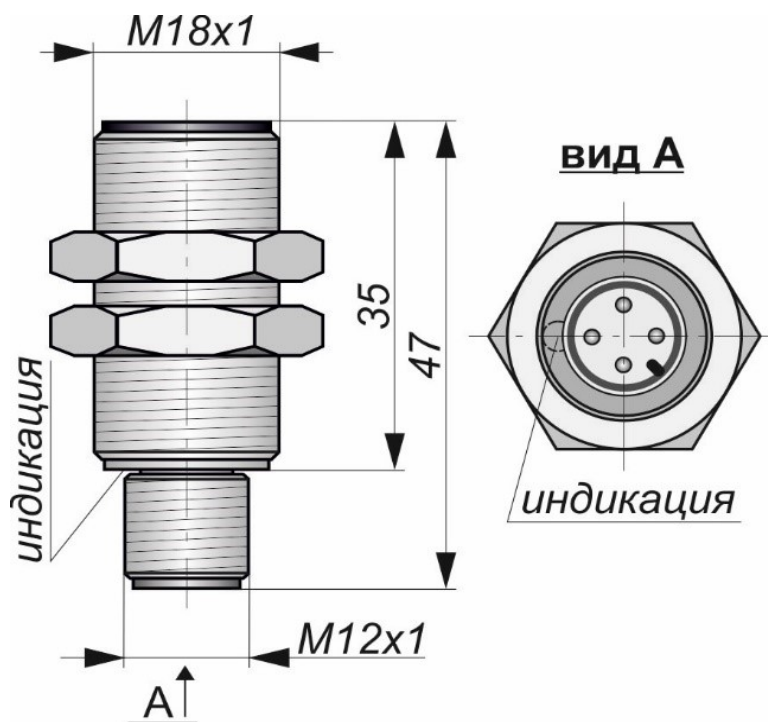
Габаритный чертеж
