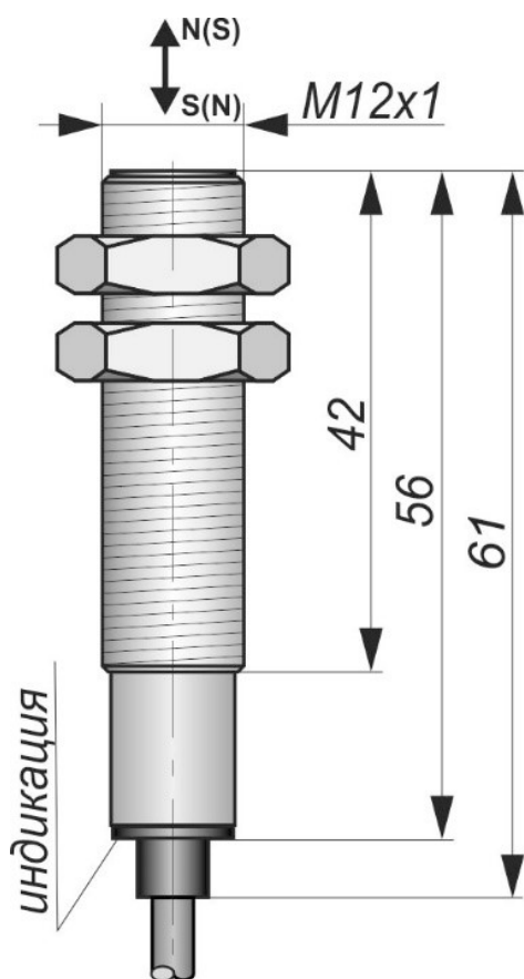
Габаритный чертеж
