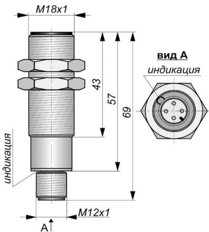
Габаритный чертеж
