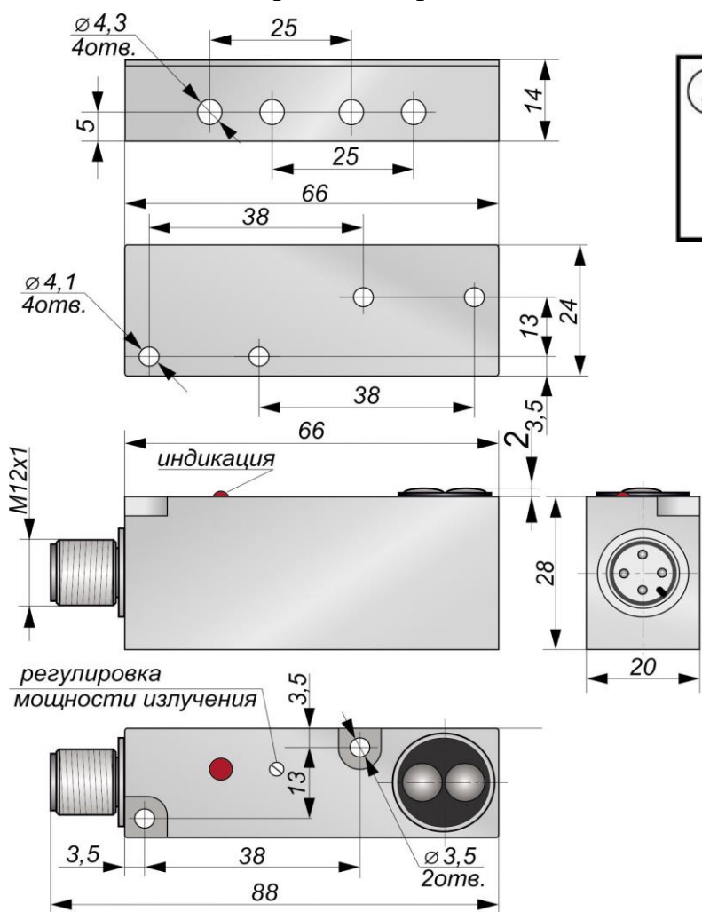
Габаритный чертеж
