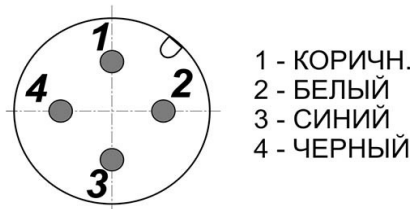
Цоколевка разъема
