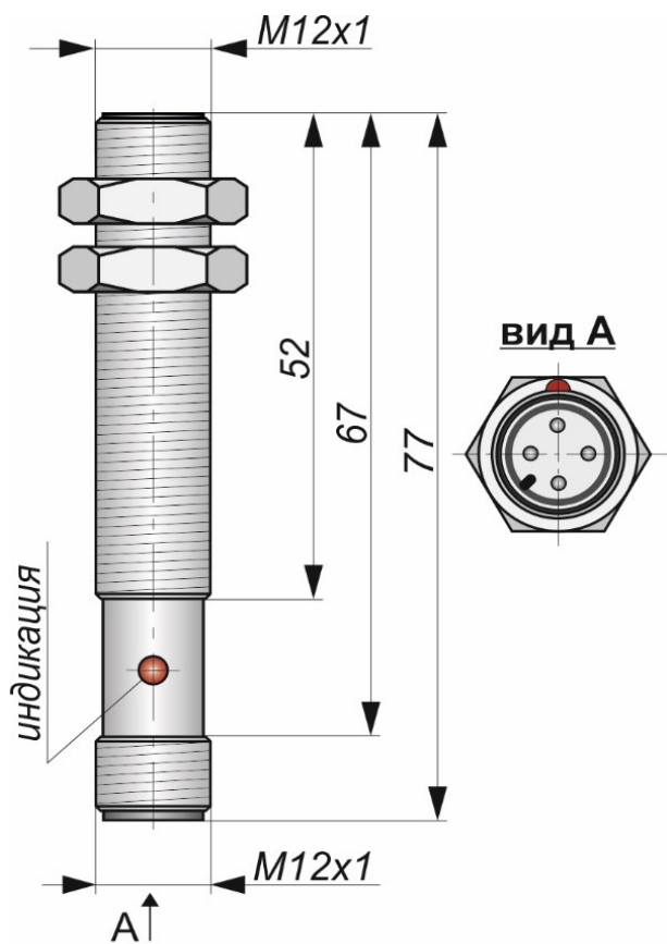
Габаритный чертеж
