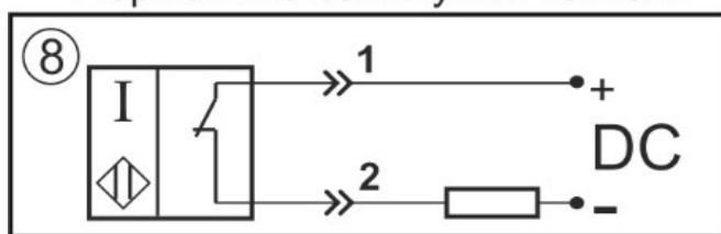
Нормально-замкнутый контакт
