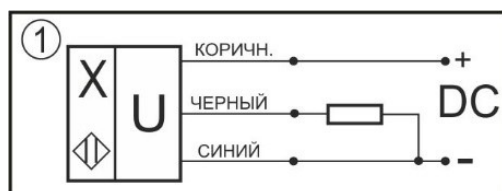
Схема соединения
