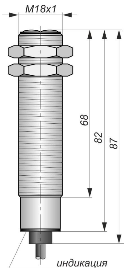
Габаритный чертеж
