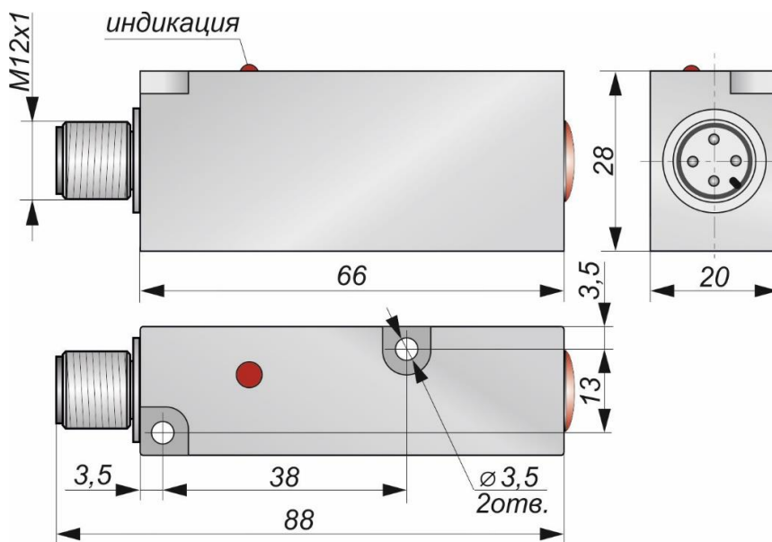
Габаритный чертеж
