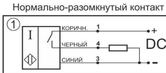
Схема соединения
