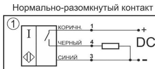
Схема соединения
