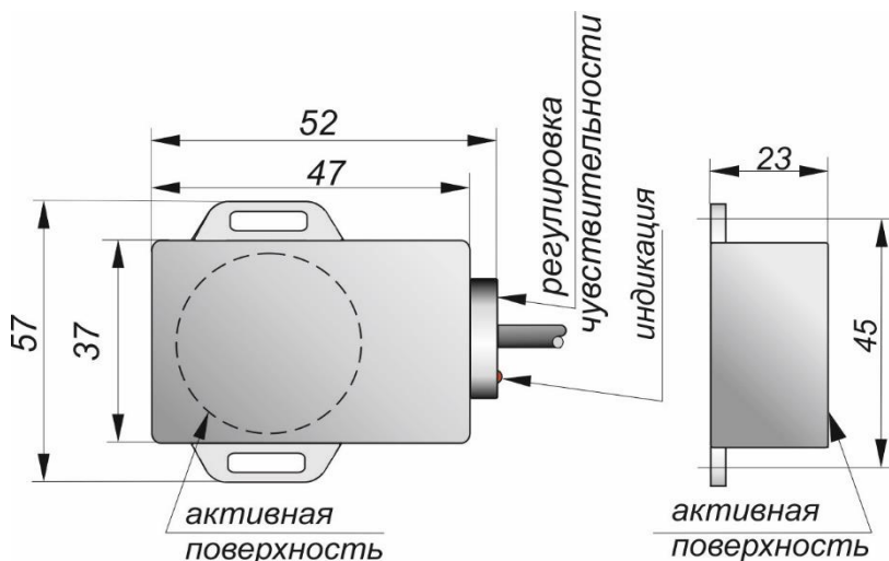
Габаритный чертеж
