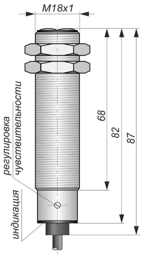
Габаритный чертеж
