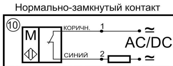
Схема подключения
