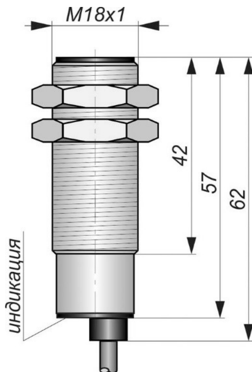
Габаритный чертеж
