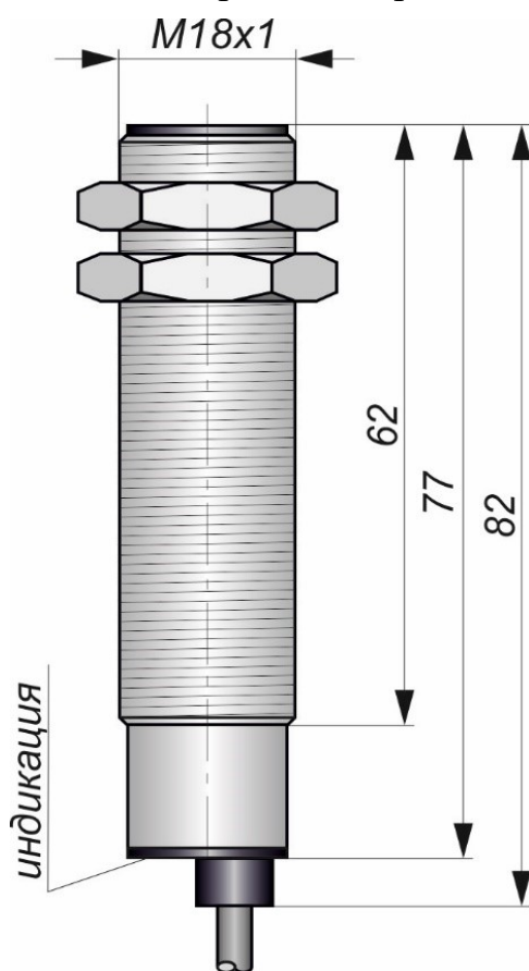
Габаритный чертеж
