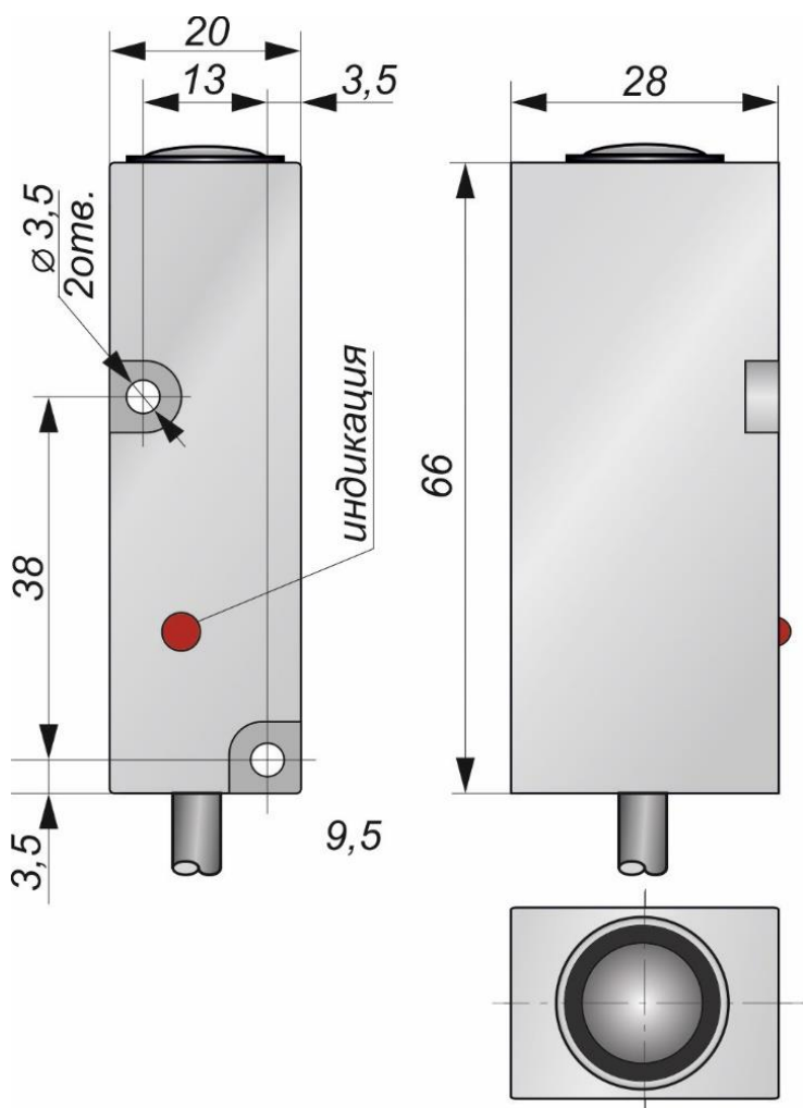
Габаритный чертеж
