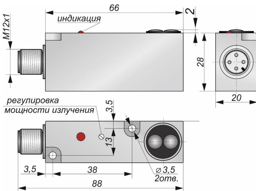
Габаритный чертеж
