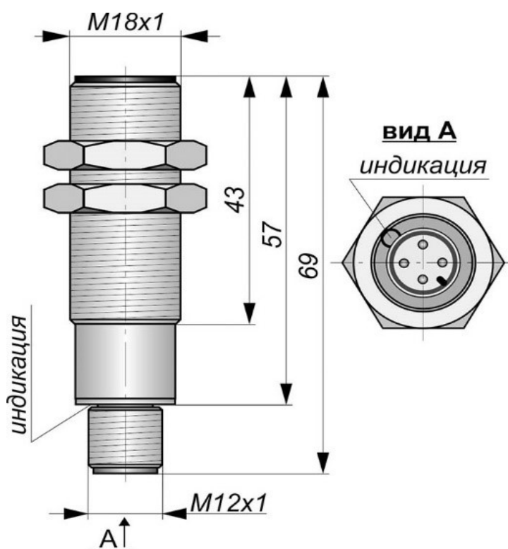
Габаритный чертеж
