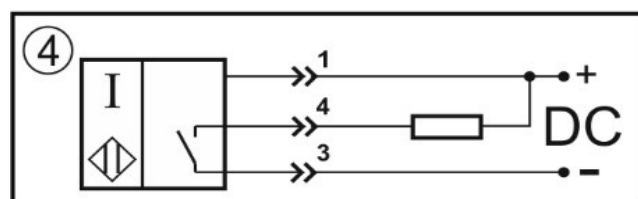
Схема соединения Нормально-разомкнутый контакт
