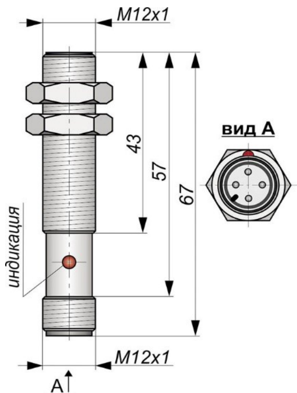
Габаритный чертеж
