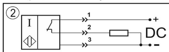
Нормально-замкнутый контакт
