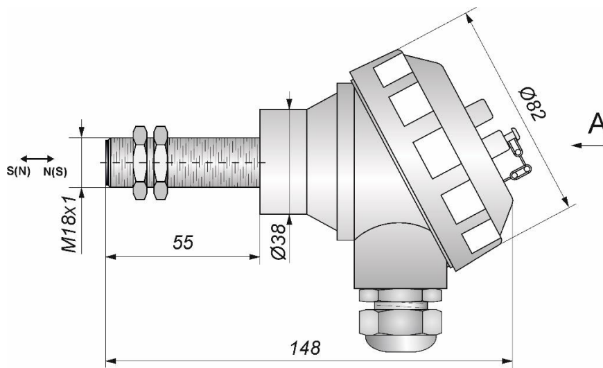
Габаритный чертеж
