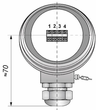
Вид со снятой крышкой
