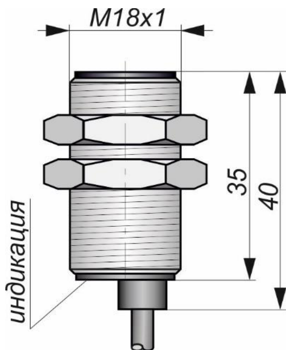
Габаритный чертеж
