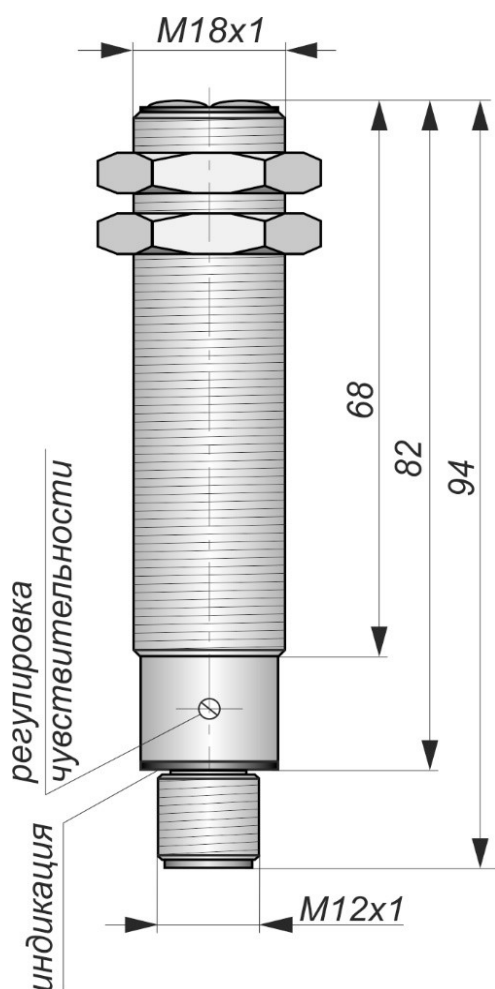
Габаритный чертеж
