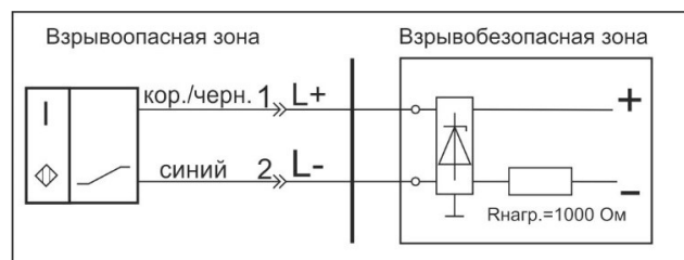
Схема соединения
