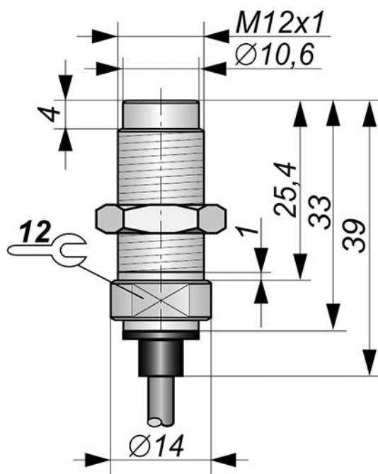
Габаритный чертеж
