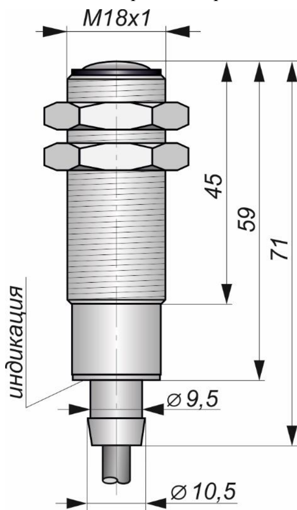
Габаритный чертеж
