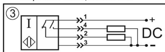
Переключающий контакт
