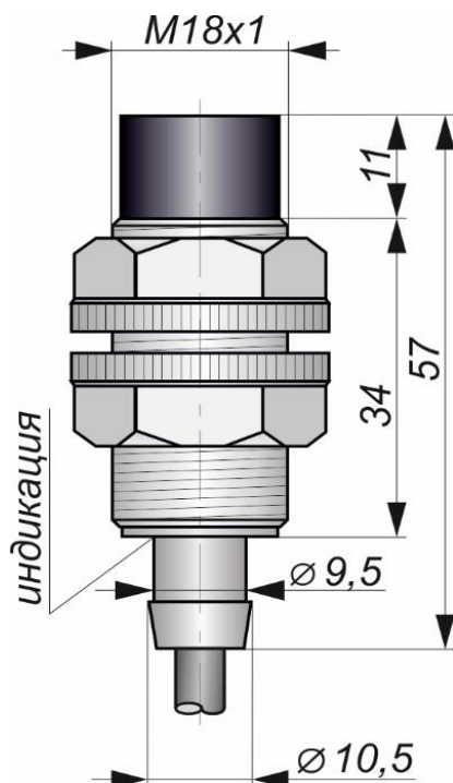
Габаритный чертеж
