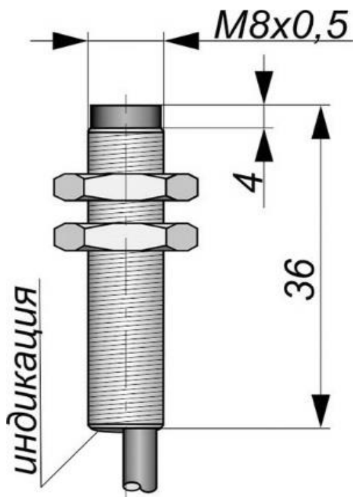
Габаритный чертеж
