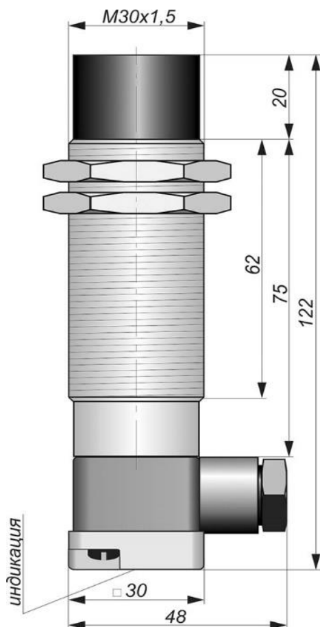
Габаритный чертеж
