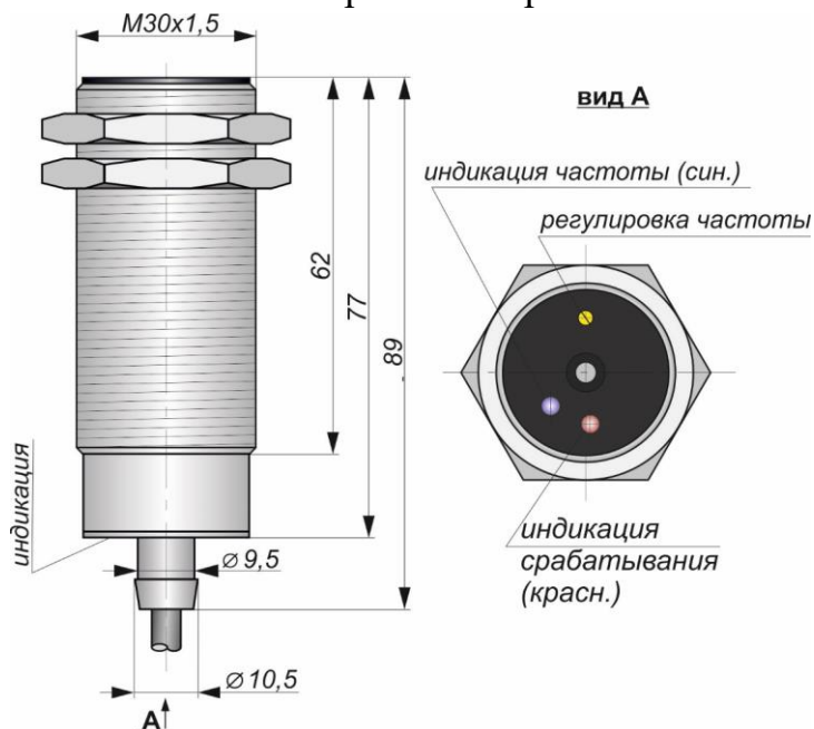
Габаритный чертеж
