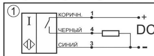
Схема соединения
