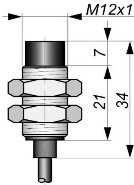
Габаритный чертеж
