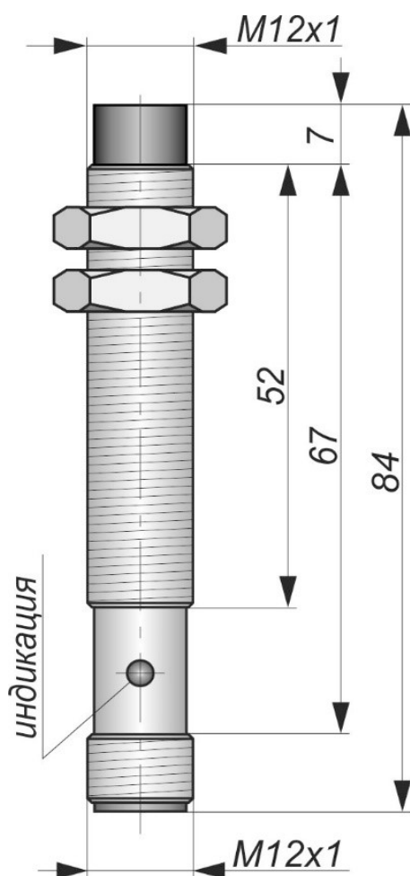
Габаритный чертеж
