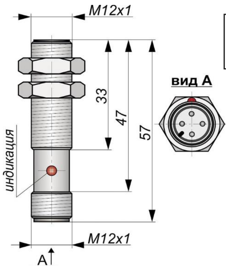
Габаритный чертеж
