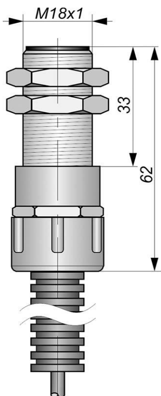
Габаритный чертеж
