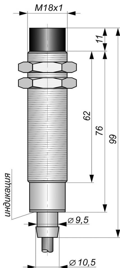
Габаритный чертеж
