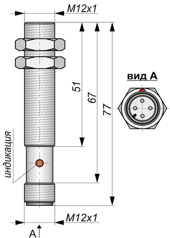
Габаритный чертеж
