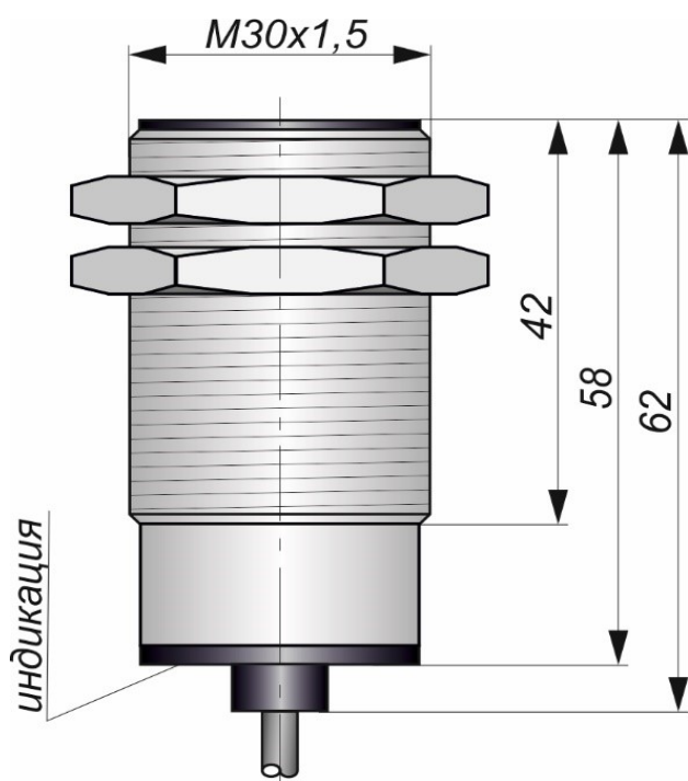
Габаритный чертеж
