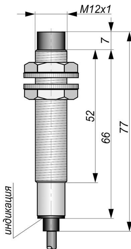
Габаритный чертеж
