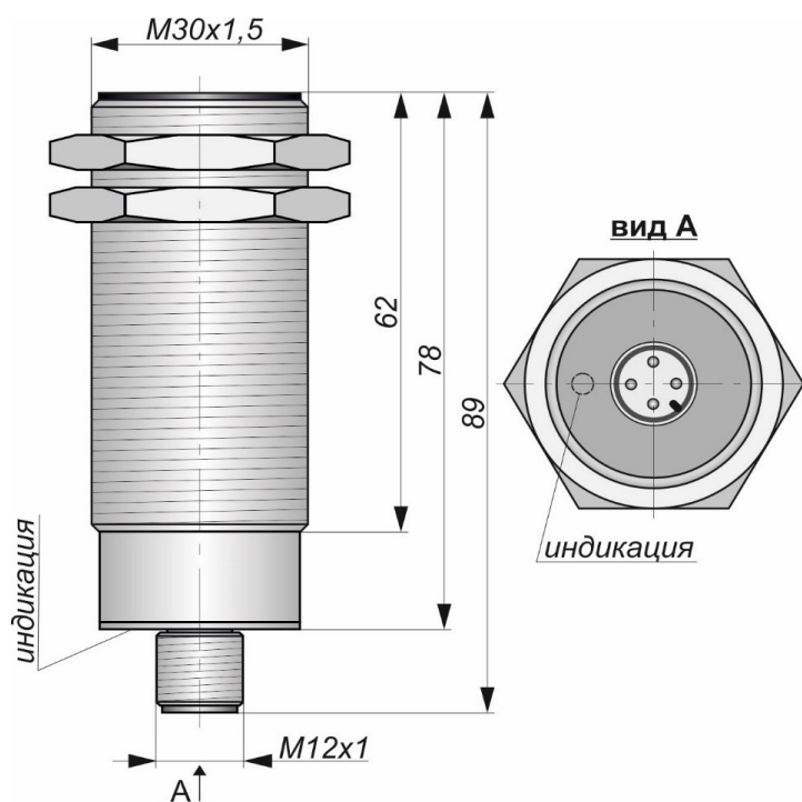
Габаритный чертеж
