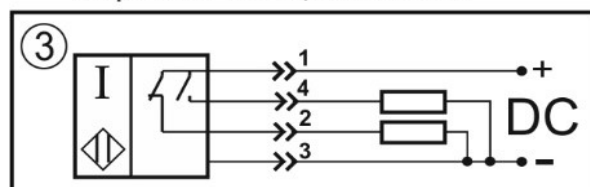
Переключающий контакт
