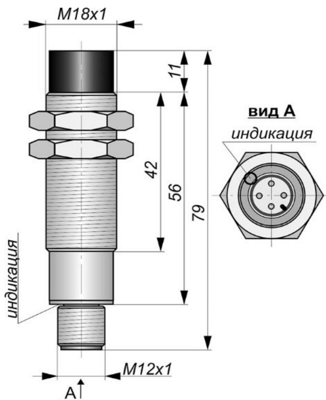
Габаритный чертеж
