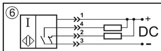
Переключающий контакт
