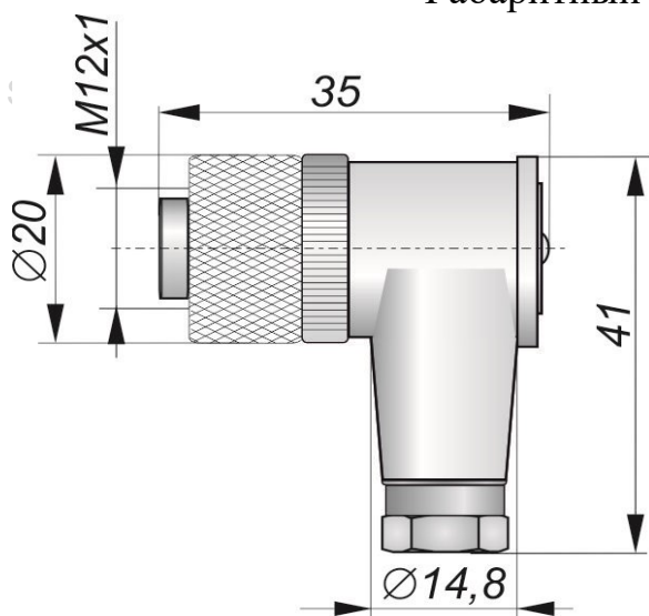
Габаритный чертеж
