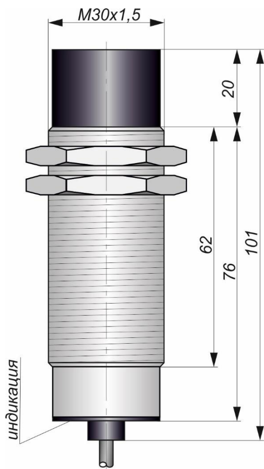
Габаритный чертеж
