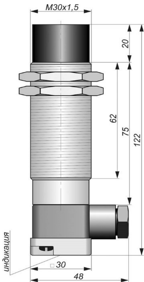
Габаритный чертеж
