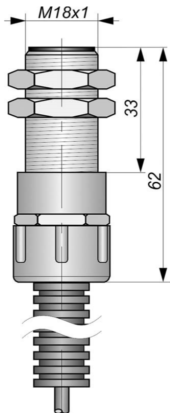
Габаритный чертеж
