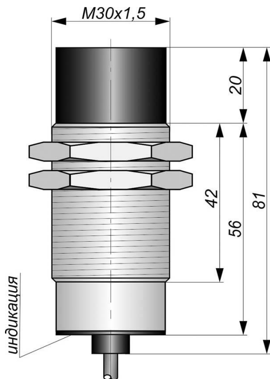
Габаритный чертеж
